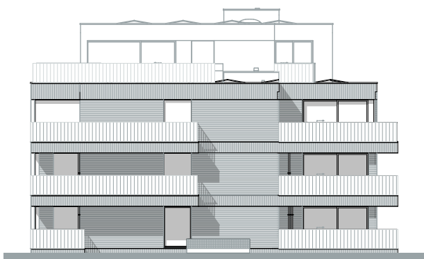
Linkergevel
